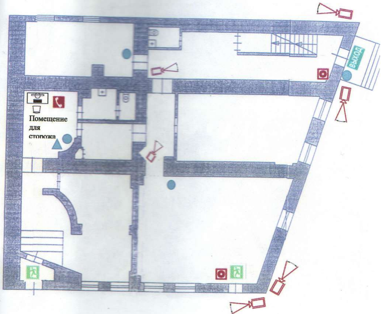
План 1 этажа. Лит. А.
